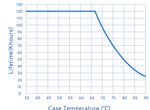
寿命Vs.壳温
