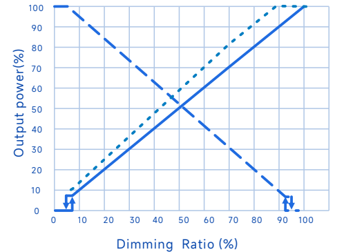
输出功率Vs.调光信号
